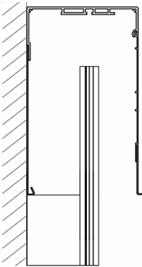
TYP A - Skrzynka pod zabudowę. Dedykowane prowadnice F-FBR-030.
